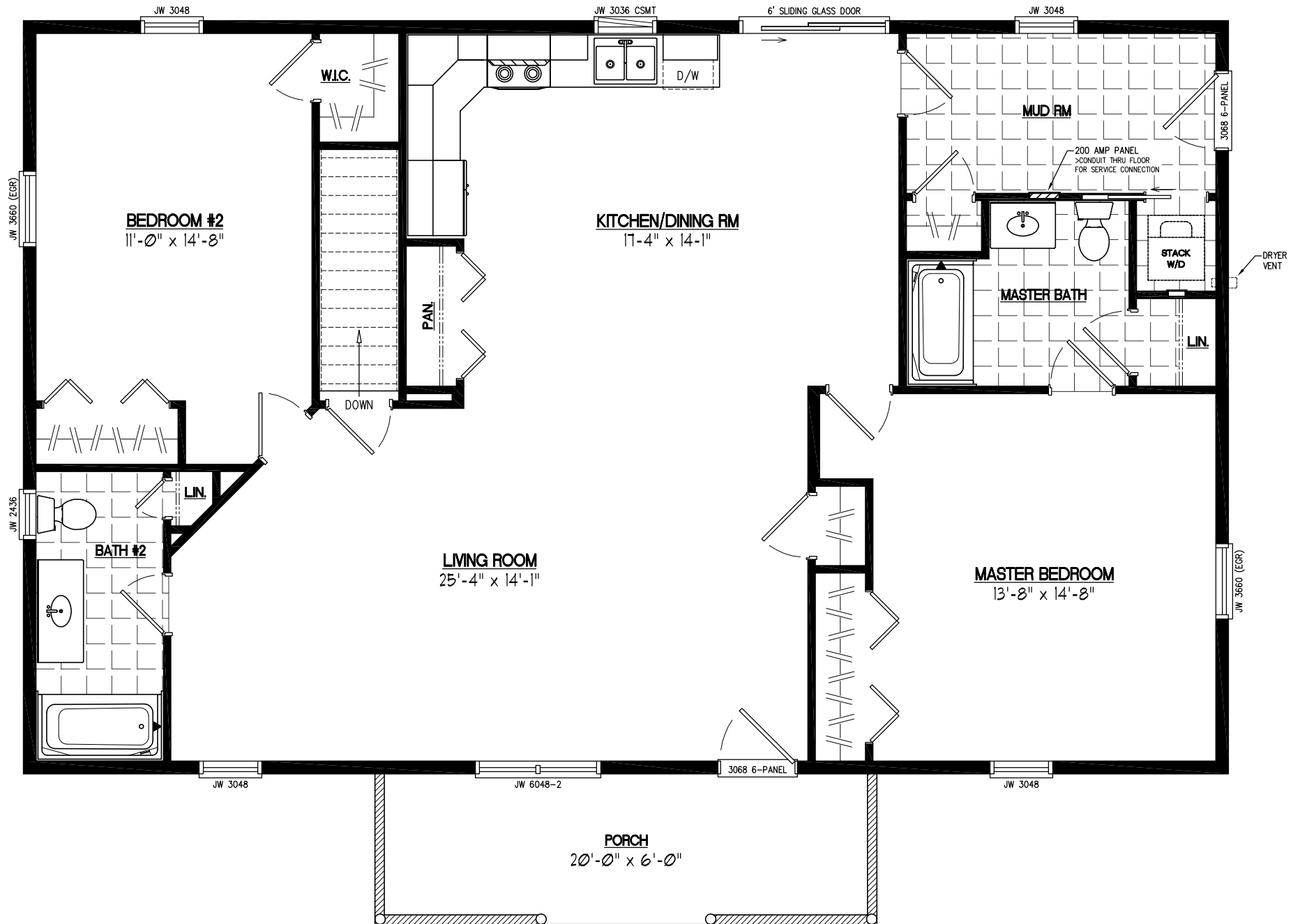
30x48 PIONEER Plan #30PR1205
