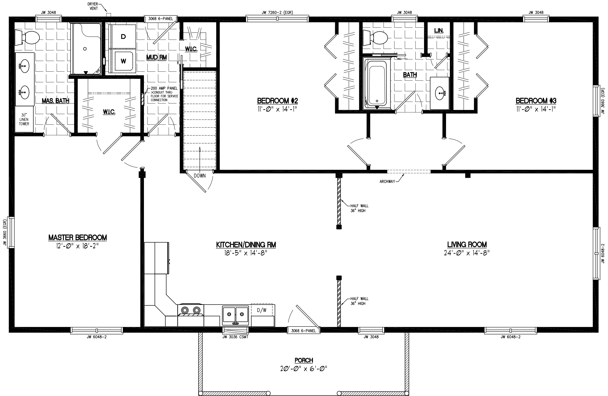
30x56 PIONEER Plan #30PR1208
